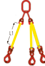
Bağlantı elemanı
