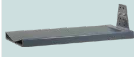
B1: V Şekilli Platform Genişlik: 247mm Uzunluk: 600mm
