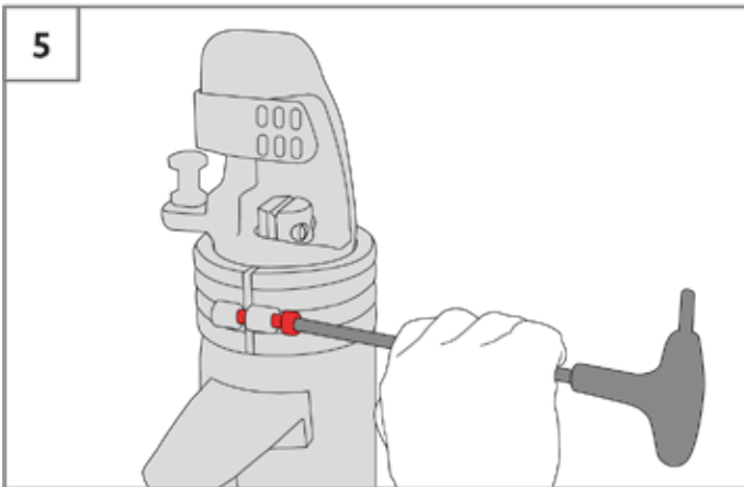
Flanşı sabitleyin
