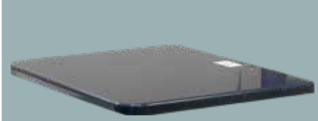
B4: Platform Üzeri Çelik Tabla PE Platform üzerinde kullanılır. Genişlik: 625mm Uzunluk: 475mm
